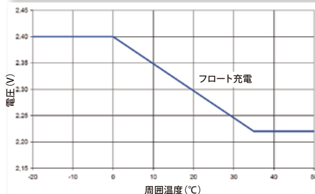
フロート充電特性 (マラソンM/FT)
