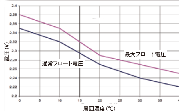
フロート充電特性 (マラソンL/XL)
